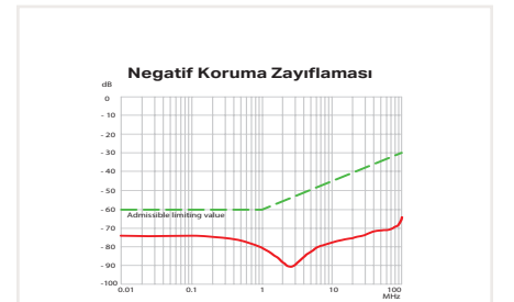
Blendaj bağlantı sistemi oldukça etkilidir çünkü sıkıştırma ünitesi kabloların blendajsız kısmına çok yaklaştırılabilir.
